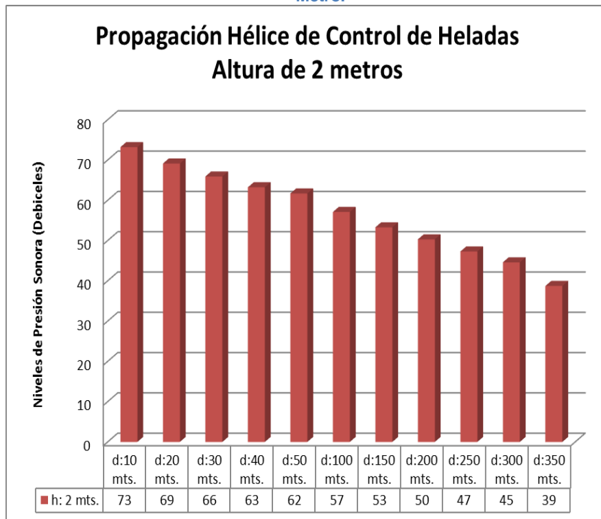
Gráfico 3: NPSeq Proyectado a Diferentes Distancias con la Hélice Portátil Funcionado a Altura de 2 Metros.
