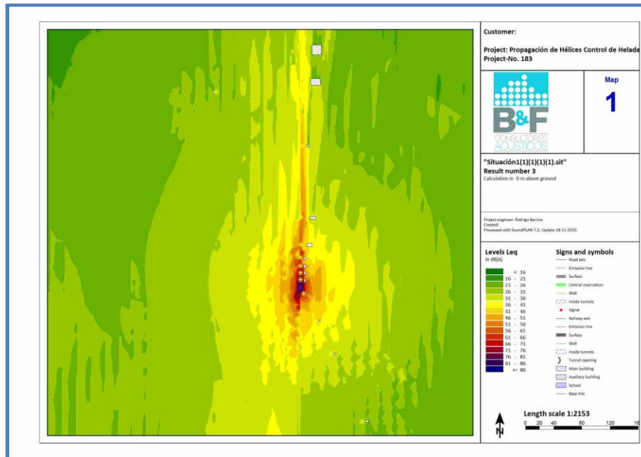
Ilustración 6: Mapa de Ruido del NPSeq Proyectado a Diferentes Distancias con la Hélice Portátil Funcionado a 7 Metros de Altura.
