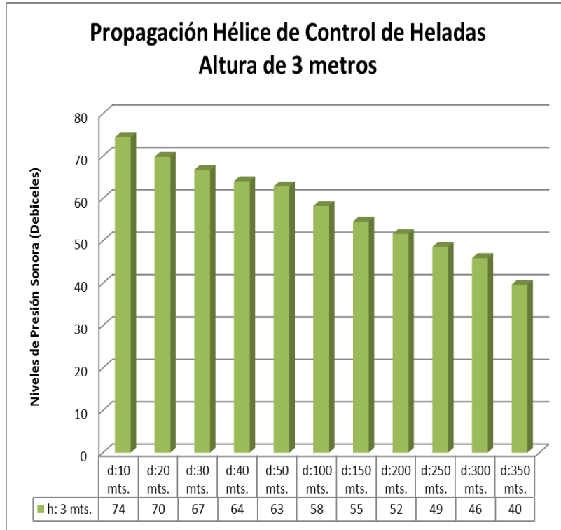
Gráfico 4: NPSeq Proyectado a Diferentes Distancias con la Hélice Portátil Funcionado a Altura de 3 Metros.
