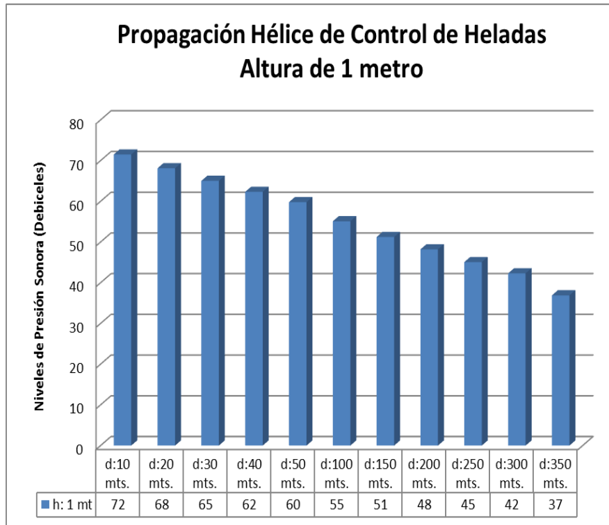
Gráfico 2: NPSeq Proyectado a Diferentes Distancias con la Hélice Portátil Funcionado a Altura de 1 Metro.
