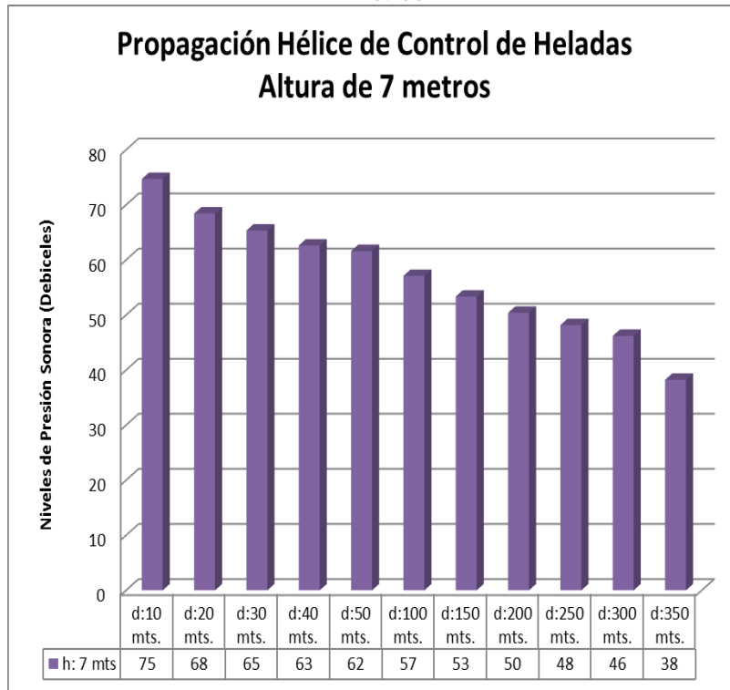
Gráfico 5: NPSeq Proyectado a Diferentes Distancias con la Hélice Portátil Funcionado a Altura de 7 Metros.
