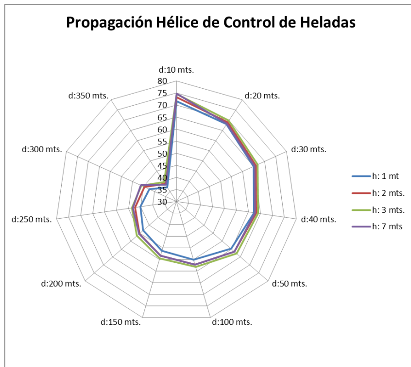
Gráfico 1: NPSeq Proyectado a Diferentes Distancias con la Hélice Portátil Funcionado a Diferentes Alturas en Metros.
