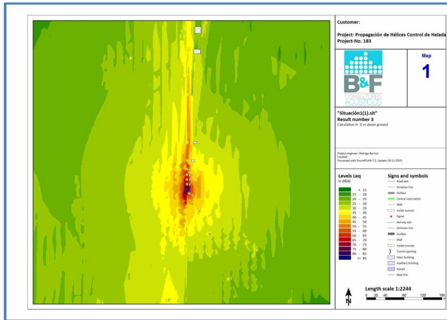
Ilustración 3: Mapa de Ruido del NPSeq Proyectado a Diferentes Distancias con la Hélice Portátil Funcionado a 1 Metro de Altura.
