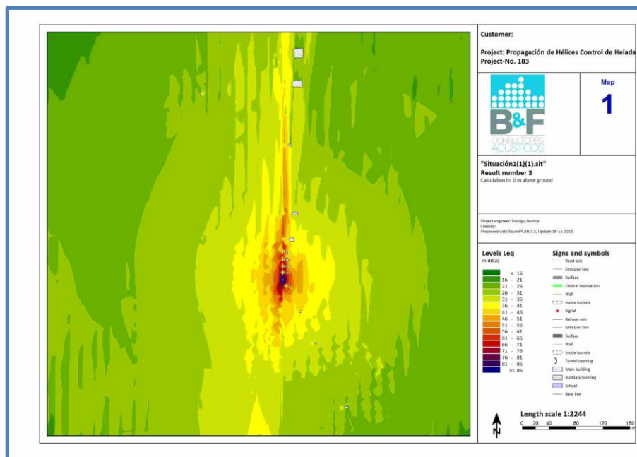
Ilustración 4: Mapa de Ruido del NPSeq Proyectado a Diferentes Distancias con la Hélice Portátil Funcionado a 2 Metros de Altura.
