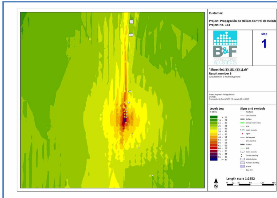
Ilustración 5: Mapa de Ruido del NPSeq Proyectado a Diferentes Distancias con la Hélice Portátil Funcionado a 3 Metros de Altura.
